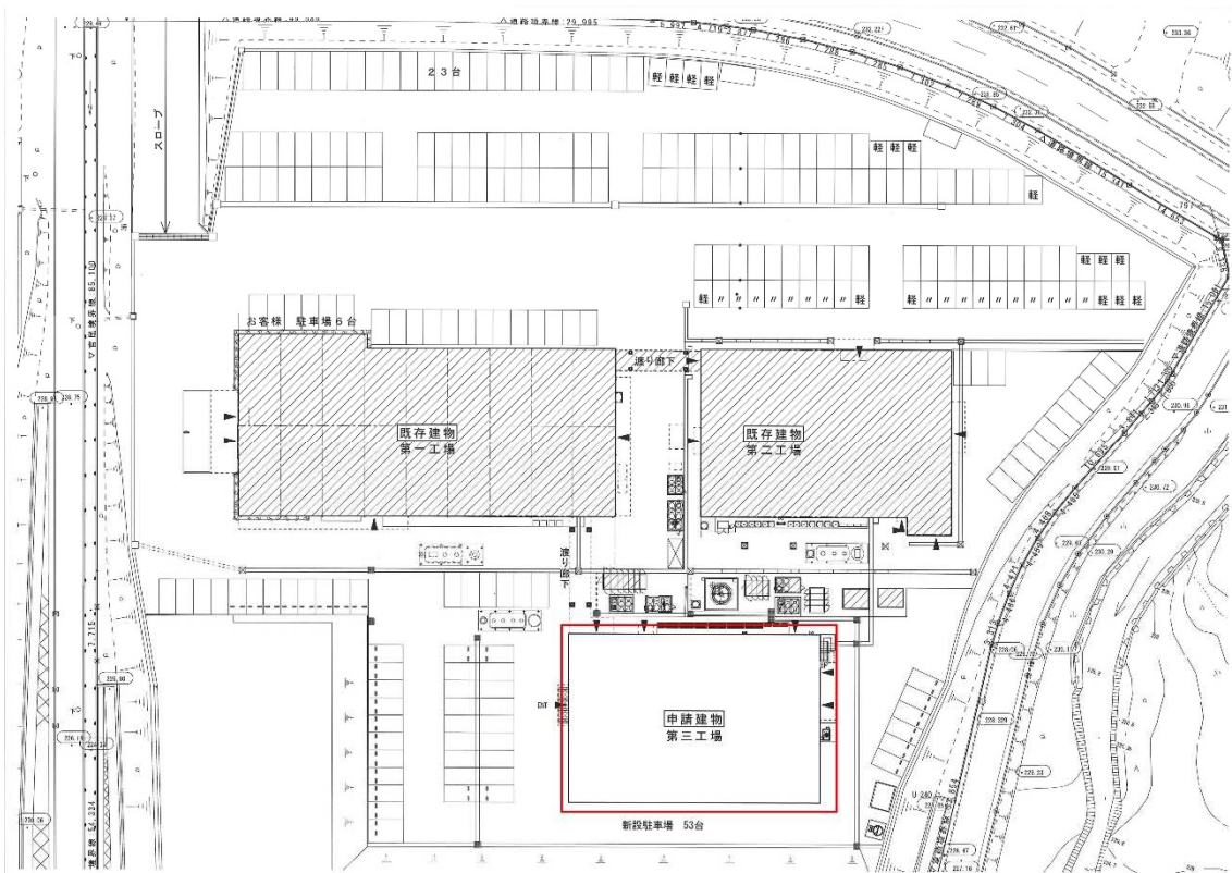
新工場配置図
